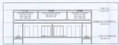
SECTION C-C SCALE: 1:100
