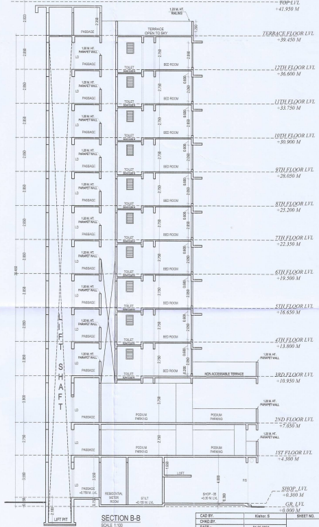
SECTION B-B SCALE: 1:100
