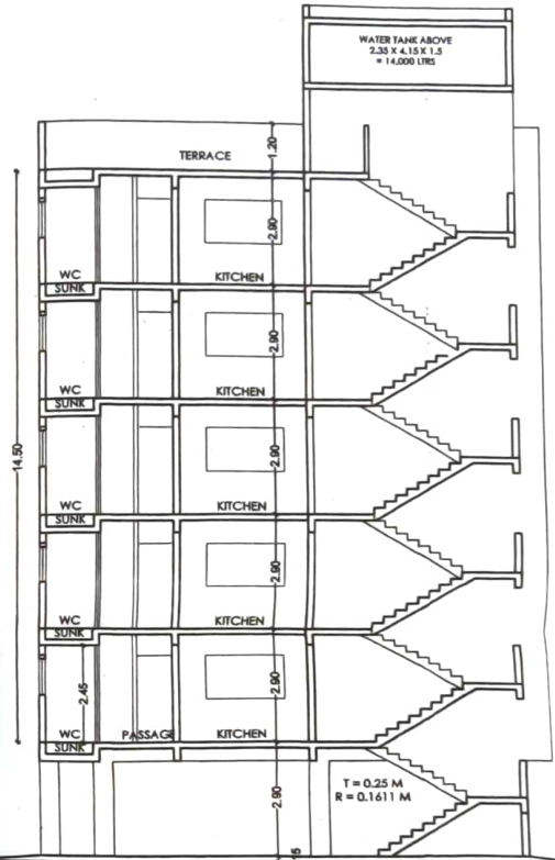
SECTION A-A
