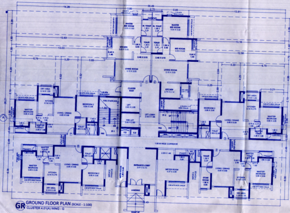
6R GROUND FLOOR PLAN (SCALE: 1:100) CLUSTER 4 (D) WING - G
