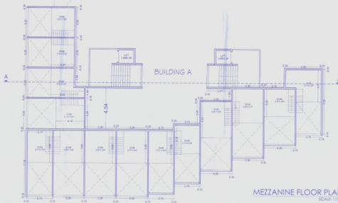
MEZZANINE FLOOR PLAN SCALE: 1:100
